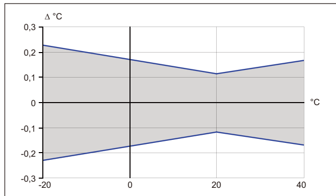
HMP155 温度測定範囲の精度
