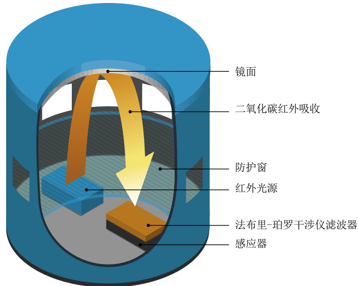
CARBOCAP传感器结构
